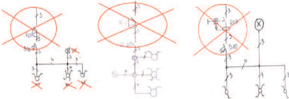
Rysunek 2. Wybrane schematy ideowe jednofazowe wykonane przez uczniów klasy III technikum elektrycznego Źródło: badania własne.
